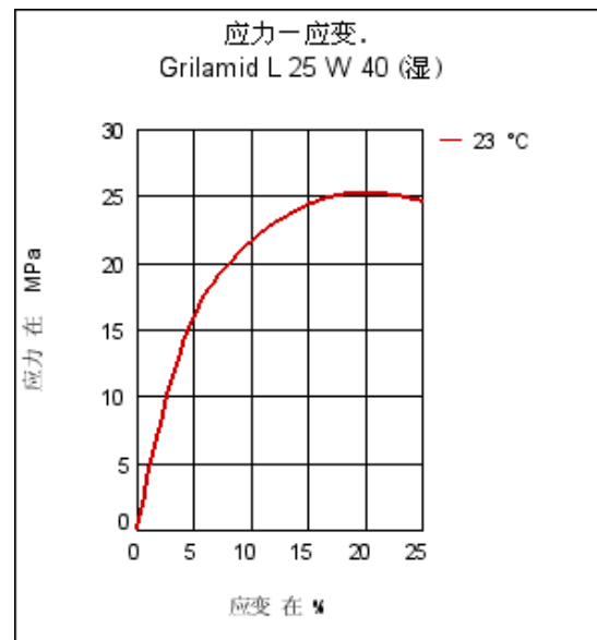
应力—应变.
